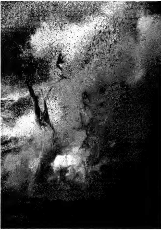
اندفاع الصحارة البركانية عبر الصدوع في قيعان المحيطات يتكون عنها الجزر البركانية
